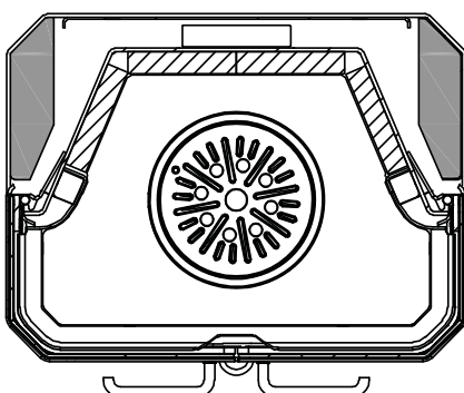
COUPE HORIZONTALE CLN
